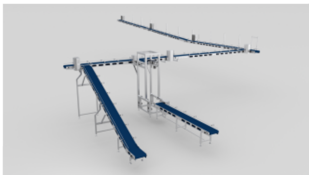
Конвейерная система с элеватором-ловератором Смотреть на сайте
